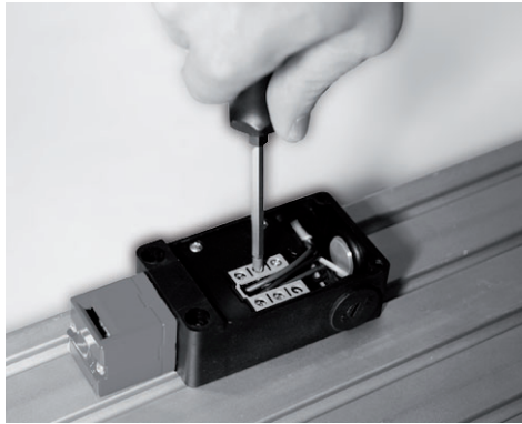
图片 7.3: 连接示范 L100-P3C3-M20-SLM24
