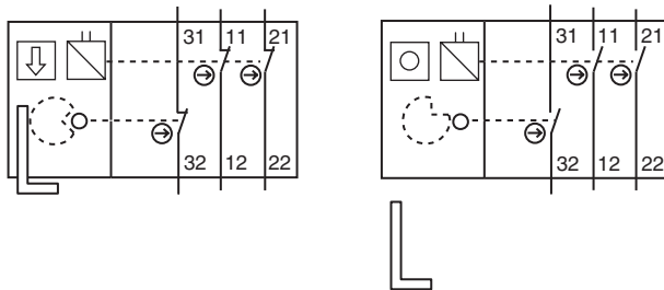
图片 7.2: 接线端子 2NC + 1NC (L100-P4C3-M20-SLM24)
