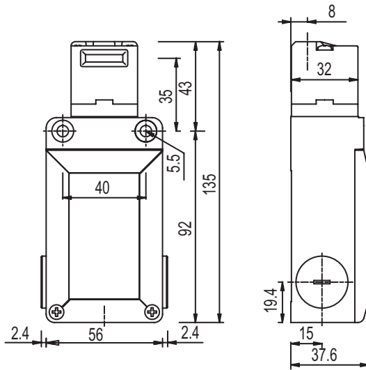
图片 3.2: L100-P3C3-M20-MLM24 的尺寸 ( mm)
