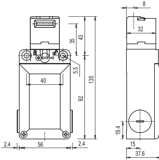
图片 3.1: L100-P3C3-M20-SLM24 和 L100-P4C3-M20-SLM24 的尺寸 ( mm)
