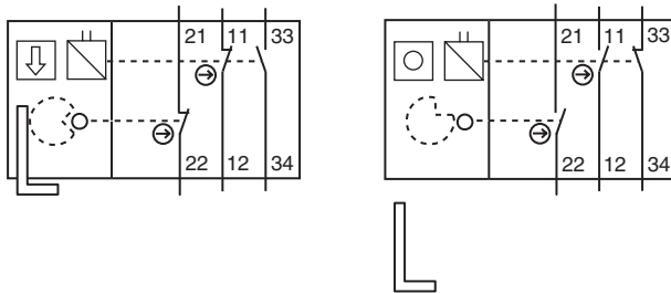
图片 7.1: 接线端子 2NC + 1NO (L100-P3C3-M20-SLM24, L100-P3C3-M20-MLM24)
