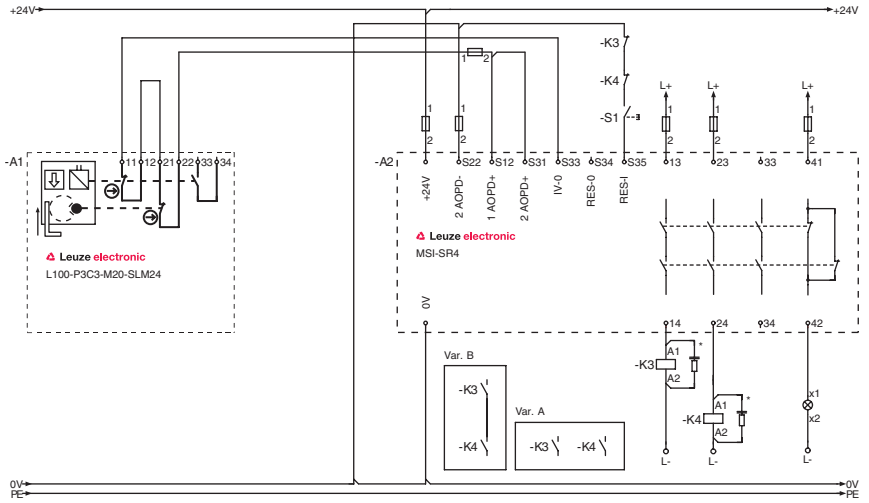
图片 7.3: 连接示范 L100-P3C3-M20-SLM24
