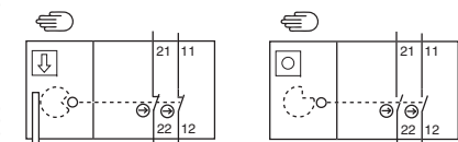
L10-P2C1-M20-SB20, L10-M2C1-M20-SB20
