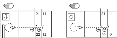
L10-P2C1-M20-SB20, L10-M2C1-M20-SB20
